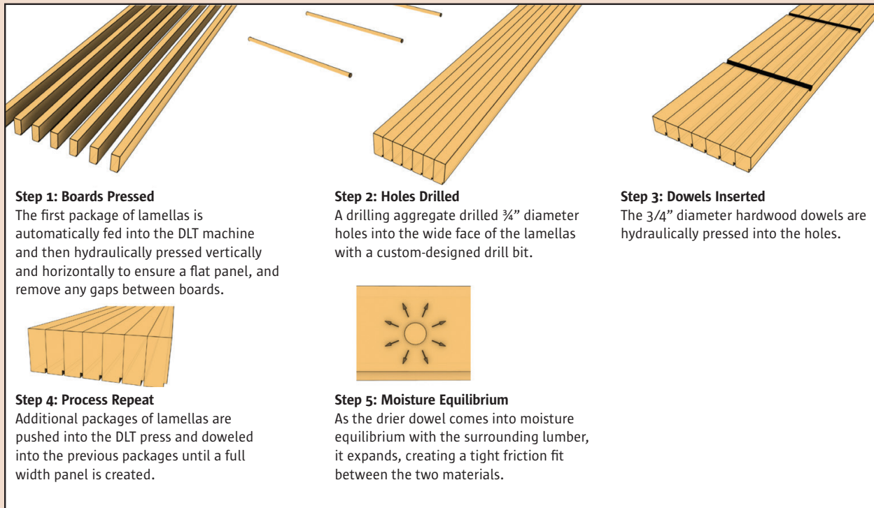
Fig. 4.12: DLT panel
